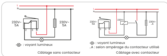
Schéma 2
