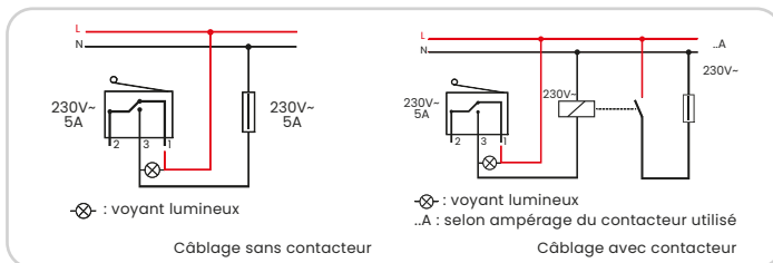
Schéma 1
